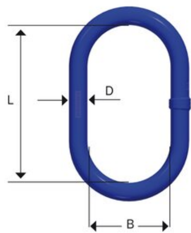
Måltabell
